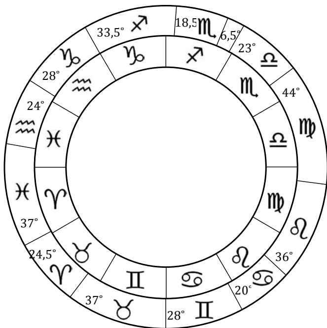
СХЕМА РАСПОЛОЖЕНИЯ ЗНАКОВ И СОЗВЕЗДИЙ
